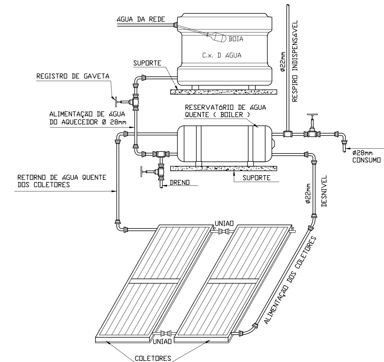
● DETALHE - AQUECIMENTO D'ÁGUA ESCALA 1:50
