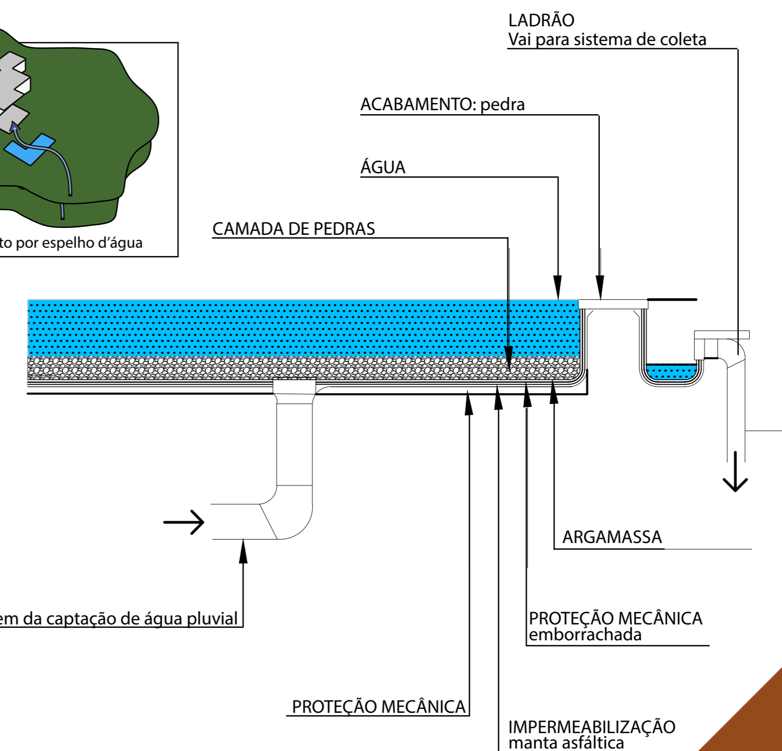
● DETALHE - ESPELHO D'ÁGUA ESCALA 1:10
