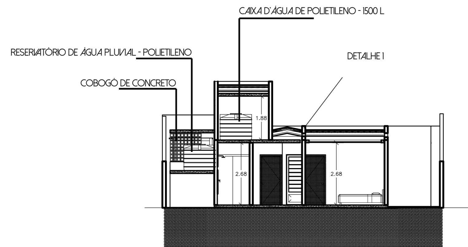
● CORTE 2 ESCALA 1:100
