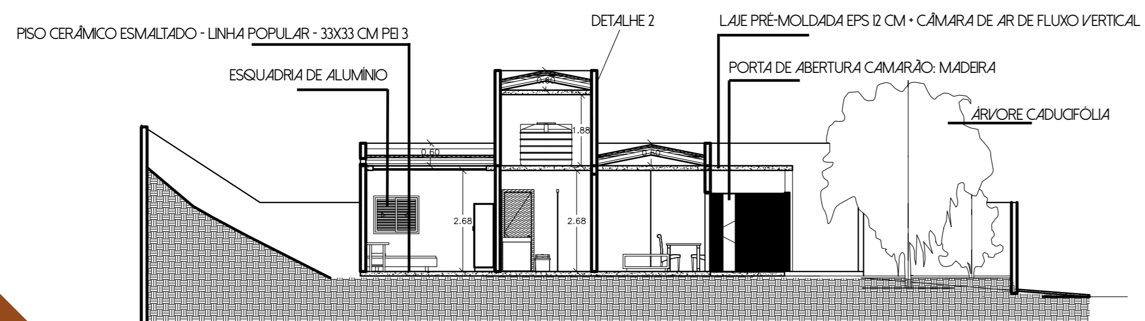
● CORTE 1 ESCALA 1:100
