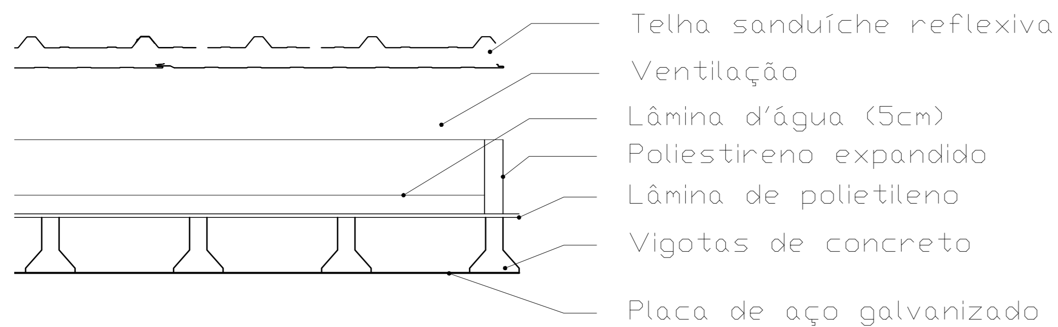
● DETALHE 1 - COBERTURA DOS QUARTOS ESCALA 1:10
